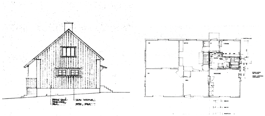
Kuva 4. Kuvassa vuoden 1994 lupakuvapiirroksia palossa vuonna 2021 tuhoutuneen asuinrakennuksen luoteis- julkisivusta sekä 1. kerroksen pohjapiirros. ©Tampereen kaupunki
